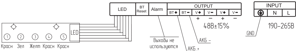
Схема подключения
